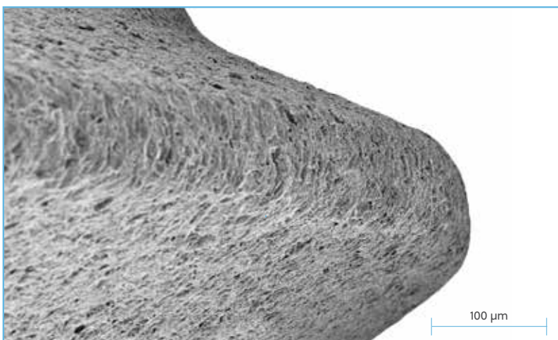
Superfície MTX num implante Tapered Screw-Vent.
